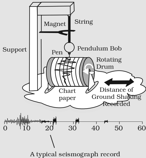
Fig. 15.13 : A seismograph
